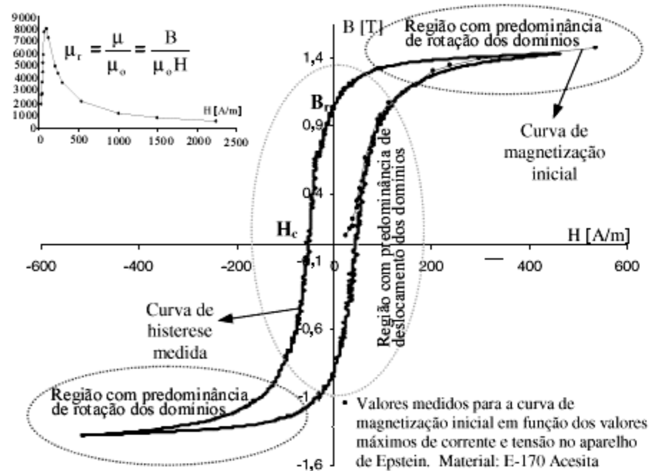
Figura 1: Curva representativa da histerese medida à 1Hz.
